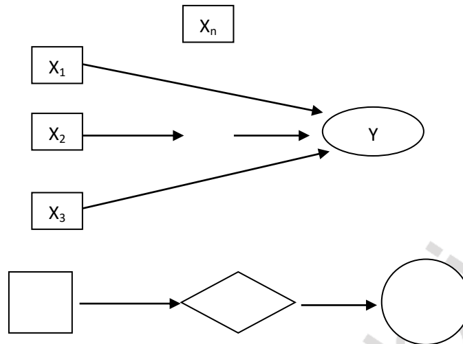
Gambar 5. Variabel pengaruh, Variabel Antara dan variabel terpengaruh
