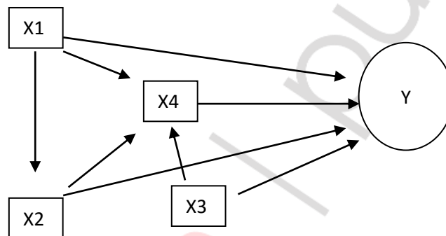
Gambar 3. Model Analisis Jalur
