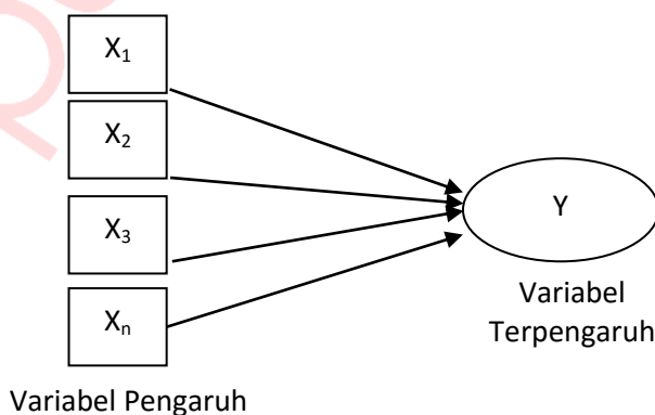
Gambar 4. Variabel Pengaruh Dan Variabel Terpengaruh
