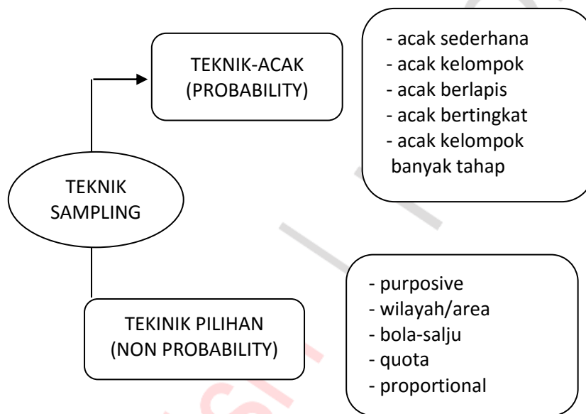
Gambar 10. Ragam Teknik Sampling
