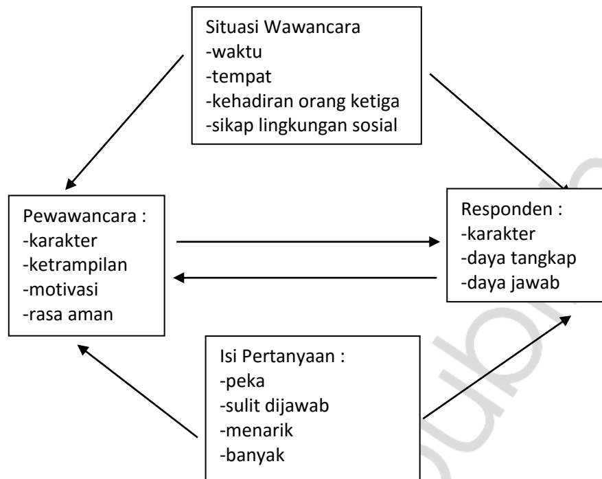
Gambar 13. Faktor-Faktor Yang Mempengaruhi Komunikasi Dalam Wawancara Tatap (Dimodifikasi)
