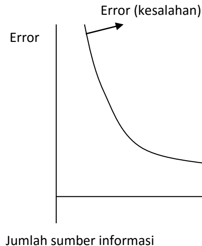
Gambar 8. Hubungan Jumlah Sumber Informasi dan Kesalahan (Error)
