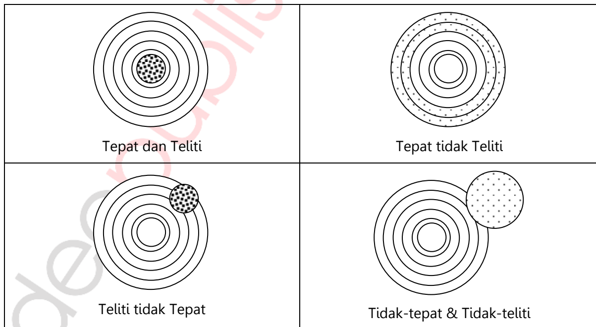
Gambar 9. Keragaman Peluang Terjadinya Ketepatan dan Ketelitian
